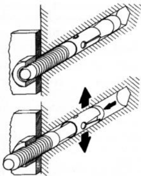
Fig. 6 - Espansione a trazione
